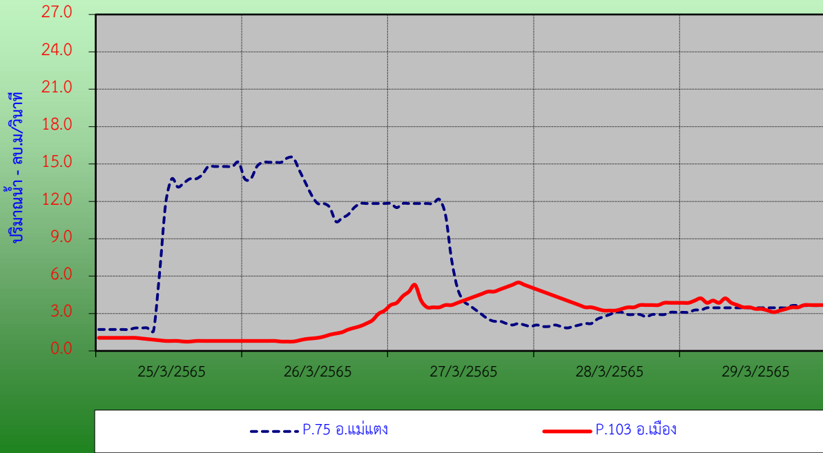
กราฟแสดงปริมาณน้ำปิ้งรายชั่วโมงรอบวันที่ 12/2565 ที่สถานีแม่ น้ำปิ้ง ( P.75) บ้านซ้อแล อ.แม่แตง และที่สถานีแม่ น้ำปิ้ง(P.103) บ้านป่าซ่อยใต้ อ.เมือง จ.เชียงใหม่
